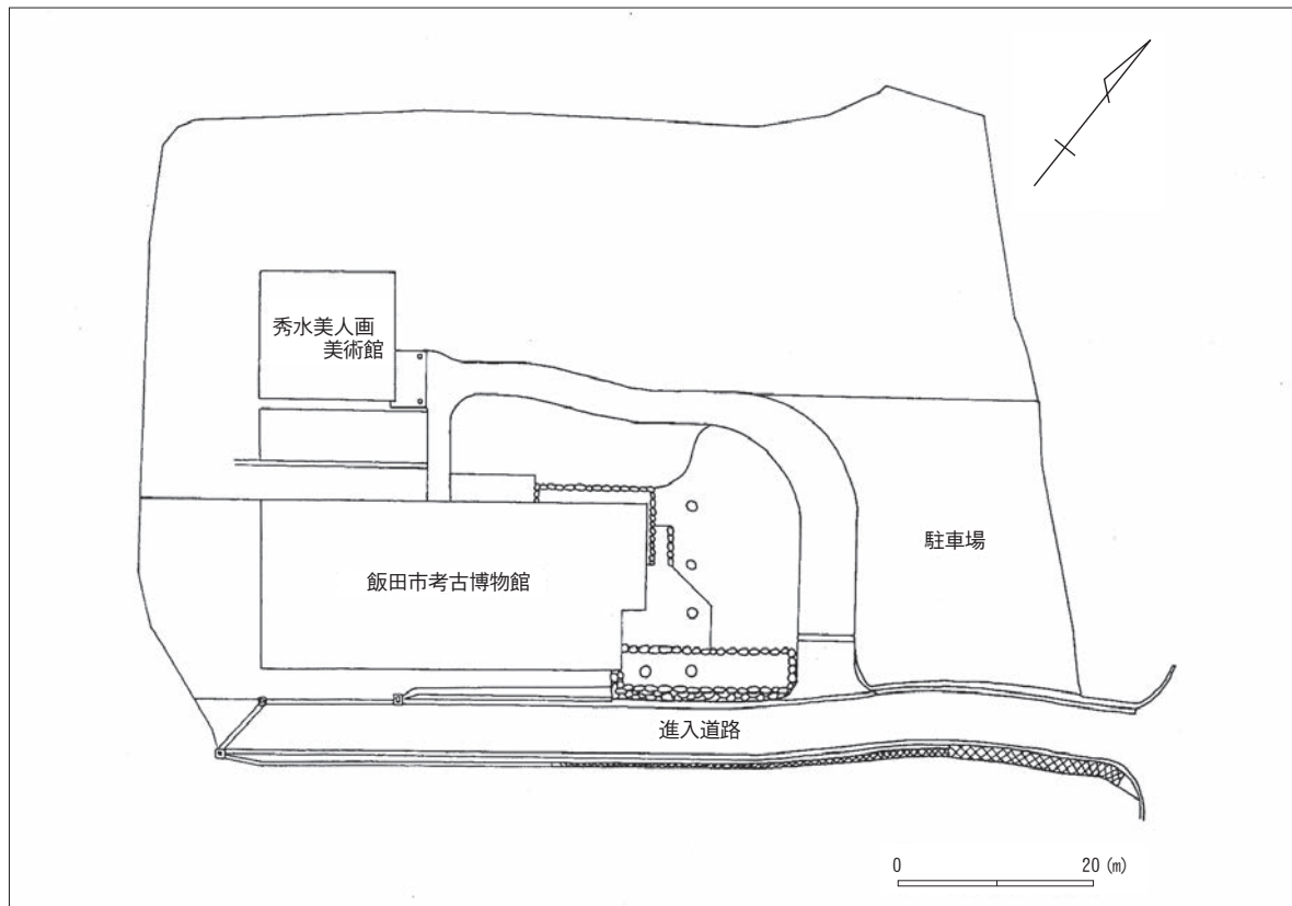
飯田市考古博物館・附属施設 平面図
